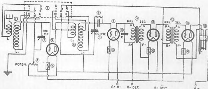
Diagrama del receptor de doble alcance. (1) Bobi na de antena; (2) conmutador para cambio de alcance; (3) Condensador variable de .001 mfd.; (4) Potenciometro de 400 ohmios; (5) primer portaválvula; (6) bobinas de inductancia; (7) condensador variables .001 mfd.; (8) condensador de rejilla de .0025 mfd. y resistencia de escape de 2 megohmios; (9) Segundo portaválvula; (10) condensador hijo de .001 mfd.; (11) primer transformador audiofrecuente; (12) tercer portaválvula; (13) segundo transformado. audiofrecuente; (14) cuarto portaválvula; (15) toma del circuito simplificado con regulador de filamento; (16) resistencias auto máticas.
